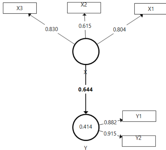
Сурет 3. Гипотезаның айнымалылар арасындағы байланыс тығыздығы
